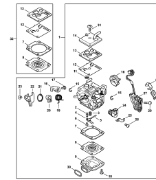
Carburetor 1142/03
