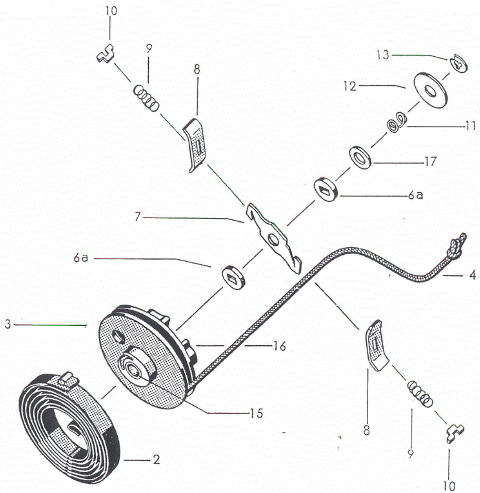
Bildtafel H Anwerfvorrichtungsteile
