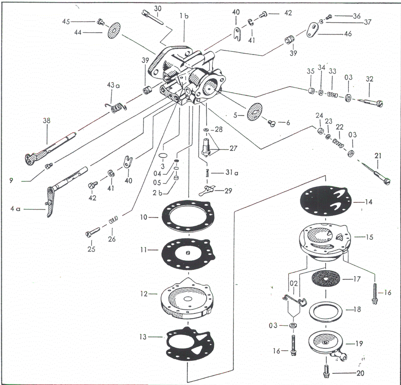
Bildtafel K Vergaser
