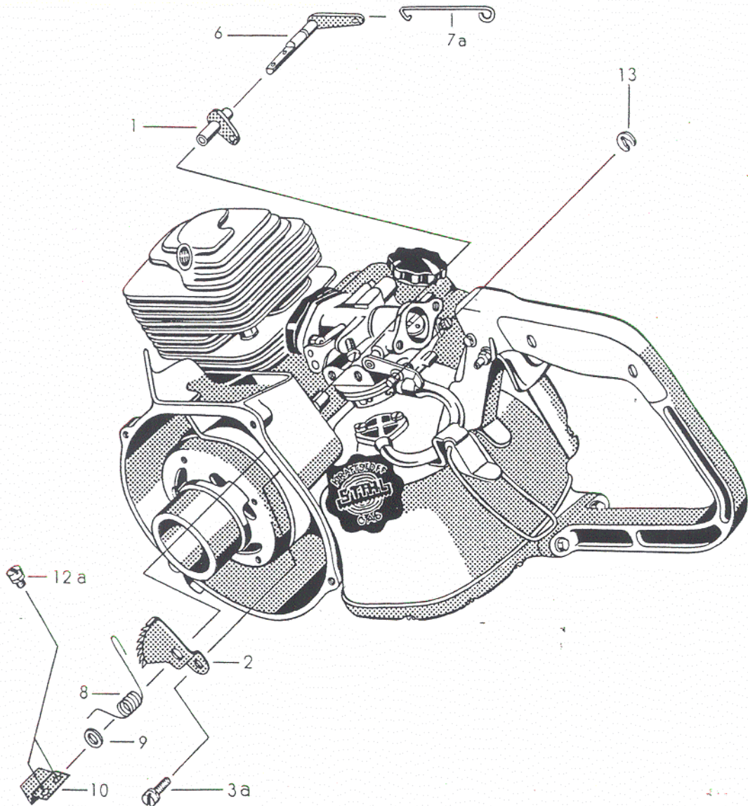
Bildtafel JJ Drehzahlbegrenzung
