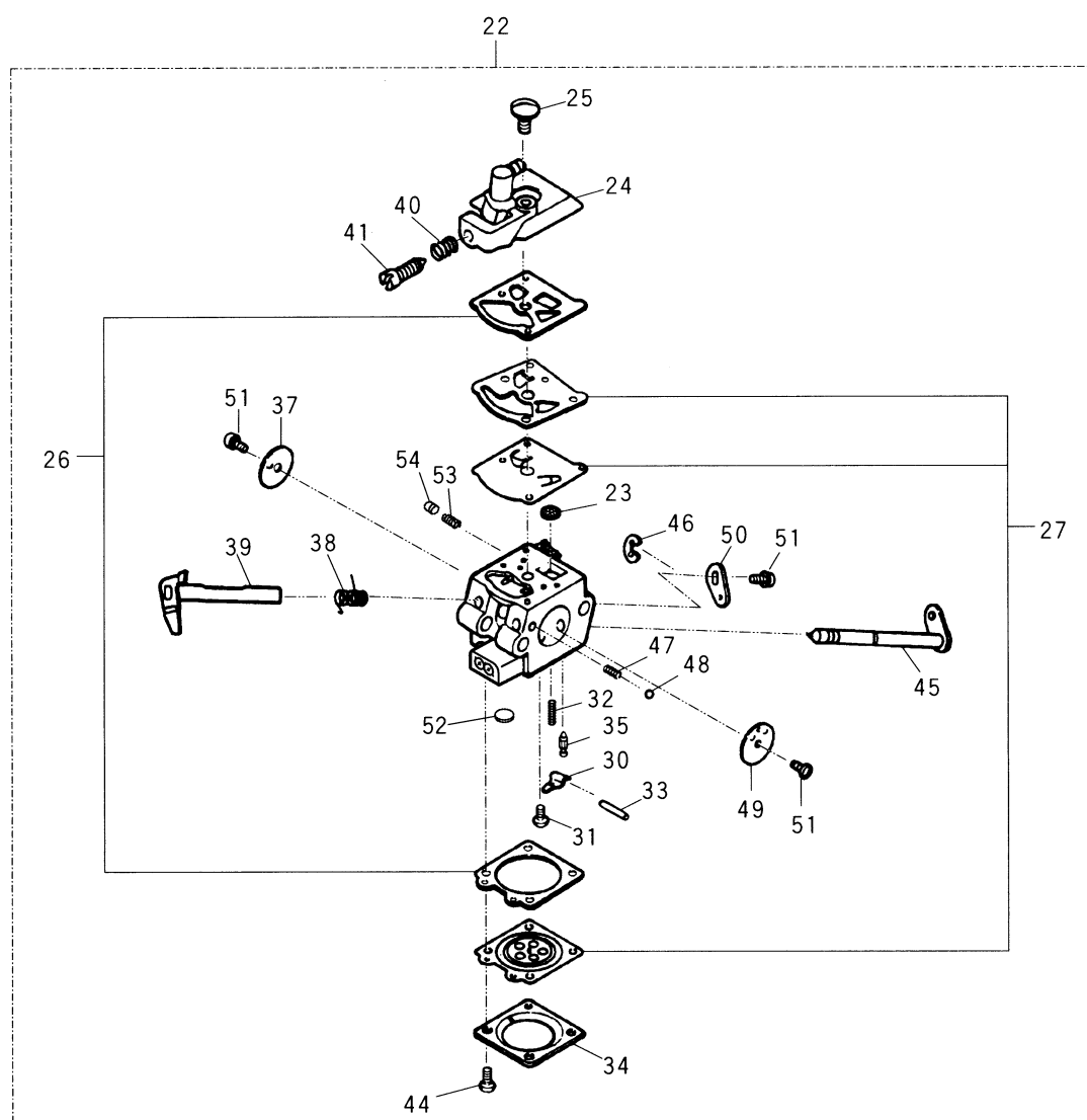
Fig.6 CARBURETOR
